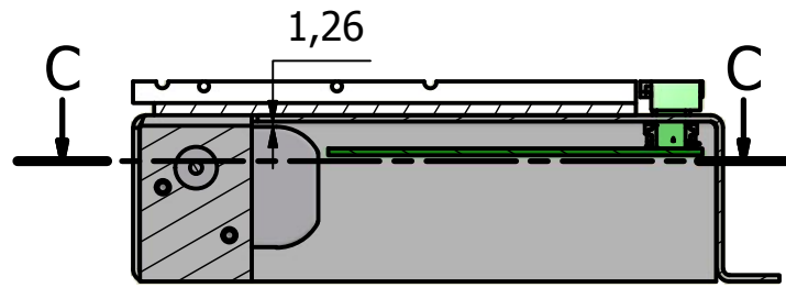
B-B ( 1 : 2 )
